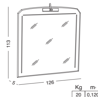
HGSS-126 SPECCHIERA 126 SAGOMATA CON FARETTO SHAPED MIRROR 126 WITH SPOTLIGHT ЗЕРКАЛО ФИГУРНОЕ 126 СО СВЕТИЛЬНИКОМ
