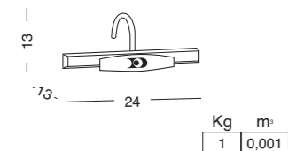
HGFA-01 FARETTO ALOGENO HALOGEN SPOTLIGHT ГАЛОГЕННЫЙ СВЕТИЛЬНИК
