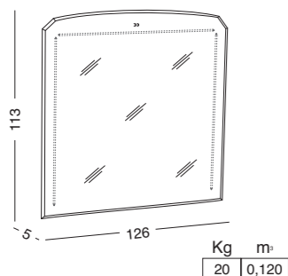
HGSL-126 SPECCHIERA 126 SAGOMATA CON LED SHAPED MIRROR 126 WITH LED LIGHTING ЗЕРКАЛО ФИГУРНОЕ 126 СО СВЕТОДИОДНОЙ ПОДСВЕТКОЙ
