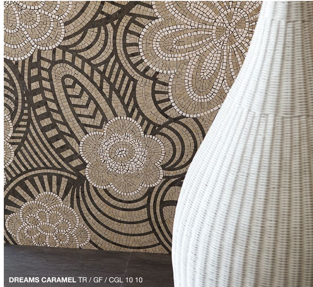
Dreams Caramel
