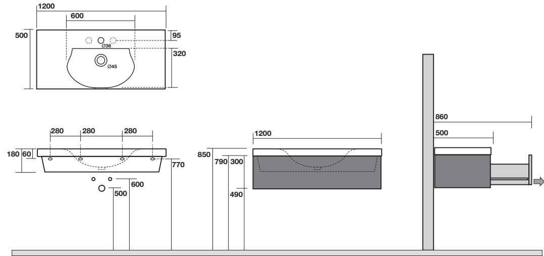
3938 Lavabo 120x50 monoforo (3 fori a richiesta) per mobile sospeso One hole washbasin 120x50 (3 holes on demand ) for cabinet 9176 Mobile sospeso in legno 120x50X30 per lavabo sospeso Wooden draw unit for washbasin 120x50X30
