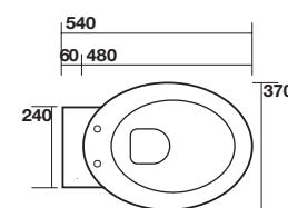
3515 Vaso ovale sospeso completo di protezione acustica e antiurto Oval wall hung wc, sound and shock proof plate included
