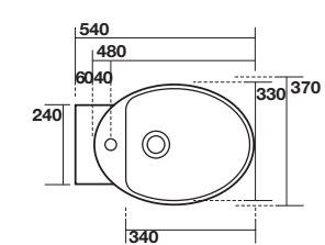
3525 Bidet ovale sospeso monoforo completo di protezione acustica e antiurto Oval one hole wall hung bidet, sound and shock proof plate included
