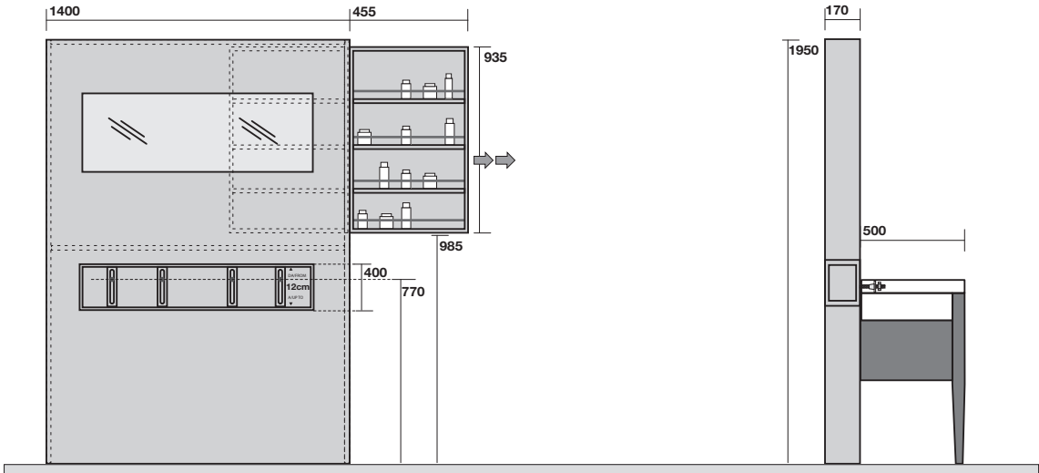
9172K Mobile pannello in legno 140x195x17 con estraibile e struttura di fissaggio per lavabo Wooden unit 140x195x17 w/hideaway shelves and metal brackets for wasbasin
