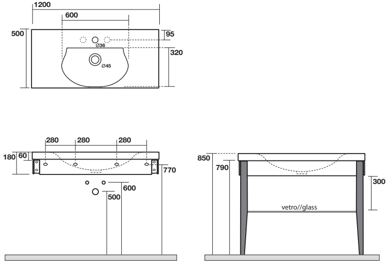
3932 Lavabo 120x50 monoforo (3 fori a richiesta) (per l'istallazione è necessaria 1 coppia di gambe in legno) One hole washbasin 120x50 (3 holes on demand) (2 wooden legs are necessary for the installation)
