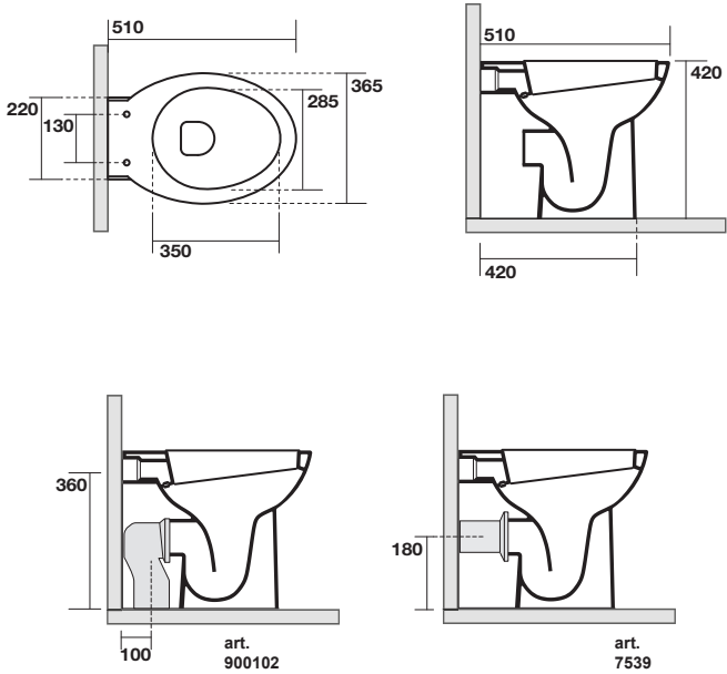
4416 Vaso unico Btw wc pan
