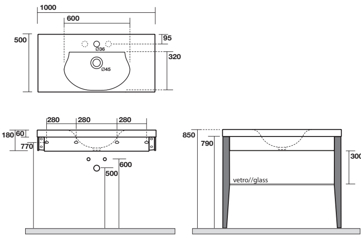
3931 Lavabo 100x50 monoforo (3 fori a richiesta) (per l'istallazione è necessaria 1 coppia di gambe in legno) One hole washbasin 100x50 (3 holes on demand) (2 wooden legs are necessary for the installation)
