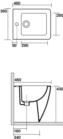
3221 bidet monoforo 46 cm completo di fissaggio WB5N Btw one hole bidet 46 cm fixing screws WB5N included
