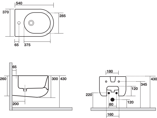
3115 Vaso sospeso completo di protezione acustica e antiurto Wall hung wc, sound and shock proof plate included
