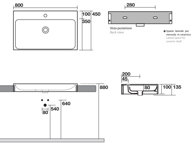
3541 Lavabo 45 Angolo sospeso o appoggio monoforo Wall hung or counter top corner basin 45 cm
