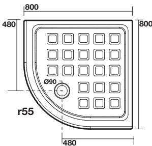
1342 Piatto doccia semicircolare 80x80 Corner shower-tray 80x80
