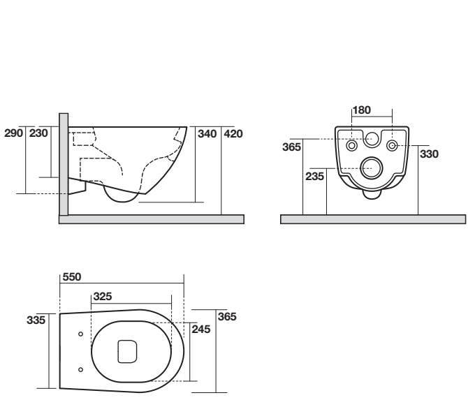
3715 Vaso sospeso completo di protezione acustica e antiurto Wall hung wc, sound and shock proof plate included
