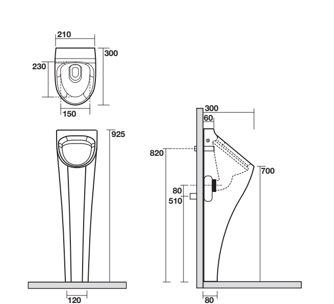
3730 Orinatoio completo di sifone e fissaggi Urinal with siphon and fixing screws
