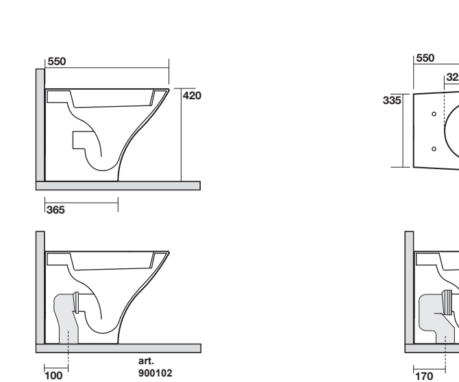
3716 Vaso unico completo di fissaggio WB5N Btw wc pan fixing screws WB5N included
