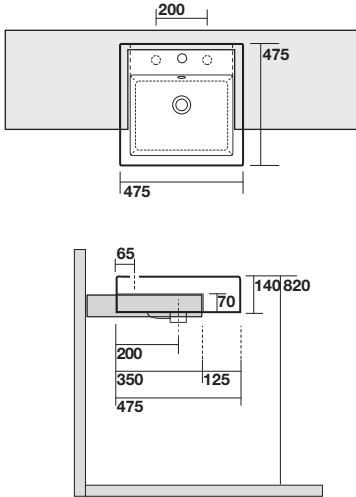
7733 “DIAMANTE” Lavabo sottopiano “DIAMANTE” undercounter basin
