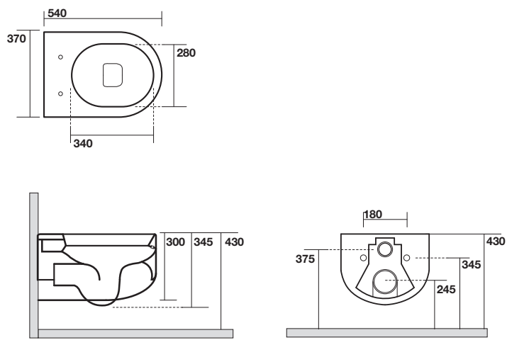
3113 vaso sospeso 54 cm completo di protezione acustica e antiurto e fissaggio WB9N Wall hung wc 54 cm, sound and shock proof plate and fixing screws WB9N included
