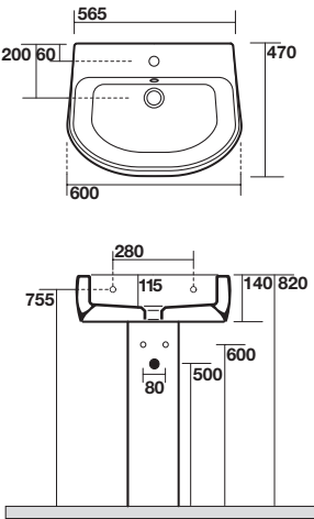
4516 Vaso unico 50 cm Btw wc pan 50 cm
