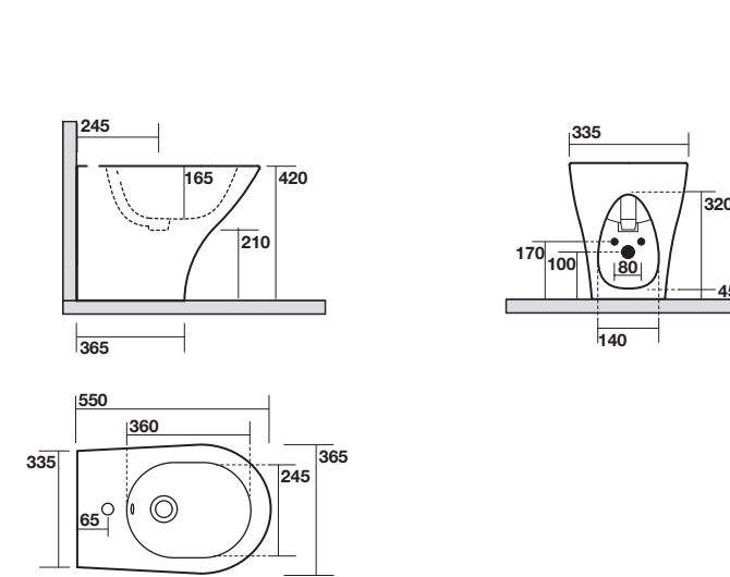
3720 Bidet monoforo completo di fissaggio WB5N Btw one hole bidet fixing screws WB5N included
