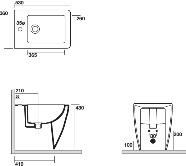
3220 bidet monoforo 53 cm completo di fissaggio WB5N Btw one hole bidet 53 cm fixing screws WB5N included
