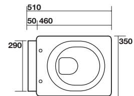
3514 Vaso rettangolare sospeso completo di protezione acustica e antiurto Rectangular wall hung wc, sound and shock proof plate included
