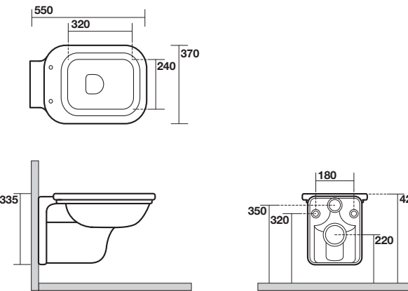
4115 Vaso sospeso completo di protezione acustica e antiurto Wall hung wc, sound and shock proof plate included
