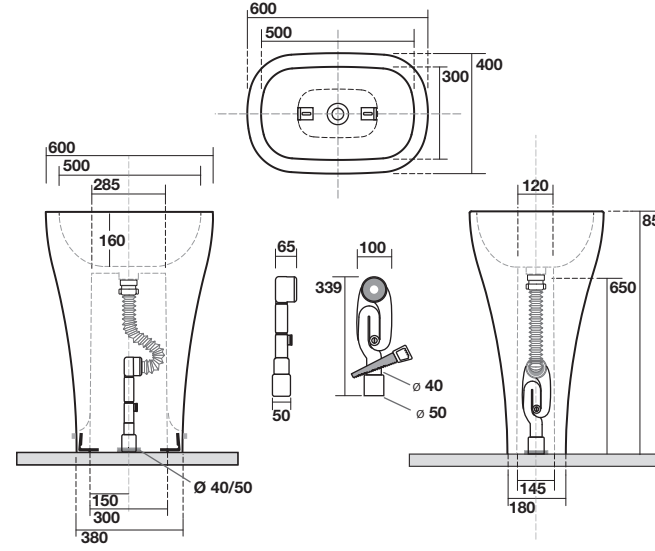
3742 Lavabo free standing 60 cm completo di fissaggio sifone e tubo flessibile di scarico One hole free-standing washbasin 60 cm siphon and flexible waste pipe included
