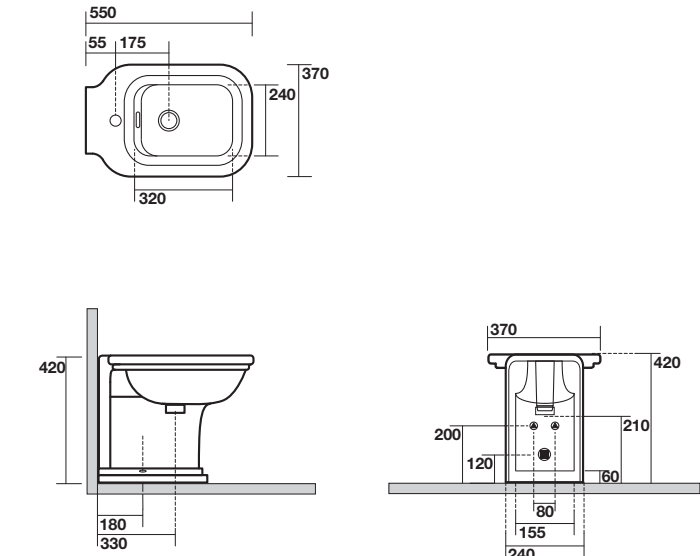
4121 Bidet monoforo Btw one hole bidet
