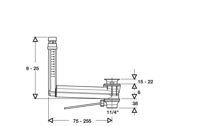
7530 Piletta con troppo pieno Drive plug w-overflow
