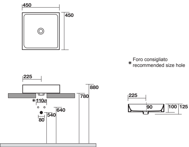
3544 Lavabo 45x45 appoggio (4 lati smaltati) Free standing washbasin 45x45 (4 glazed sides)
