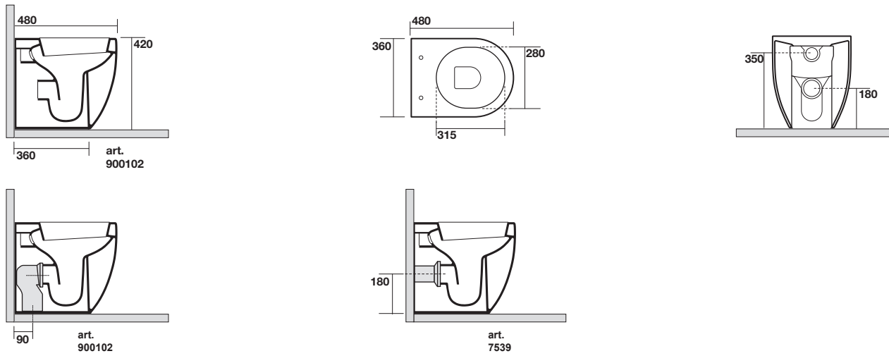
3118 Vaso unico 56 cm completo di fissaggio WB5N Btw wc pan 56 cm fixing screws WB5N included
