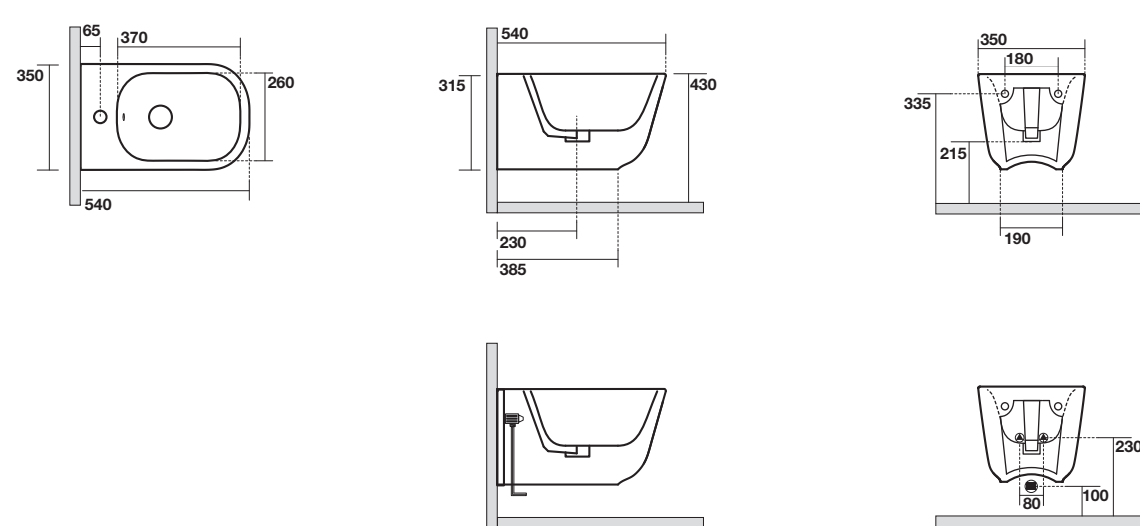
5125 Bidet sospeso monoforo completo di protezione acustica e antiurto e fissaggio WB9N One hole wall hung bidet sound and shock proof plate and fixing screws WB9N included
