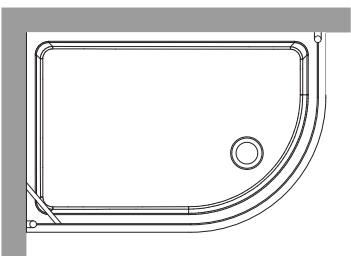
9137 Cabina doccia semicircolare DX per piatto doccia 80x120 DX. Apertura utile 63 cm, altezza 187 cm. Right semicircular shower enclosure for right shower-tray 80x120. Usable opening 63 cm, height 187 cm.
