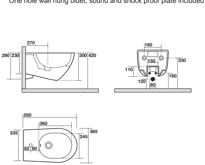
3725 Bidet sospeso monoforo completo di protezione acustica e antiurto One hole wall hung bidet, sound and shock proof plate included
