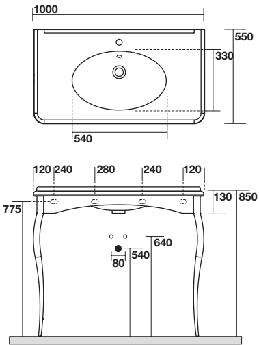
7347 Mobile chiuso per lavabo 100 Cabinet for washbasin 100
