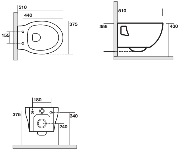
4415 Vaso sospeso Wall hung wc
