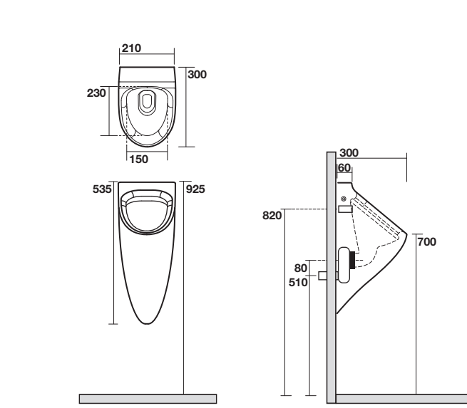
3735 Orinatoio sospeso completo di sifone e fissaggi Wall hung urinal with siphon and fixing screws
