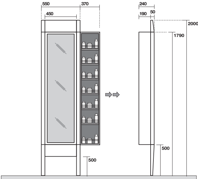
9183 Specchio a terra con contenitore estraibile 55x200x24 Mirror cabinet w/hideaway shelves 55x200x24
