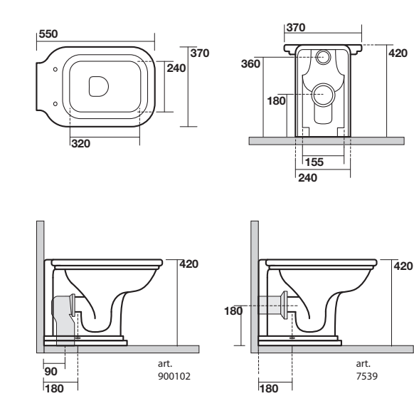
4118 Vaso unico Btw wc pan
