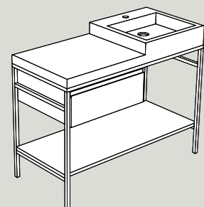
Semplice L 105 x H 83 x P 48 cm
